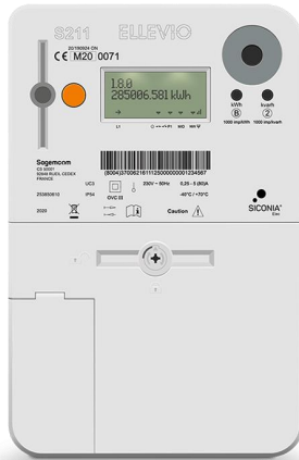
Sagemcom 1-Fas
